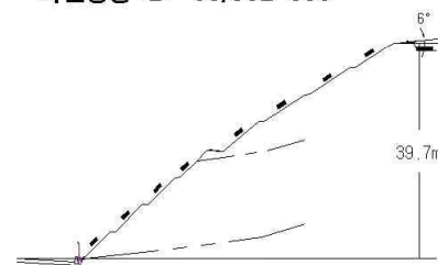
<A-A' 단면>
