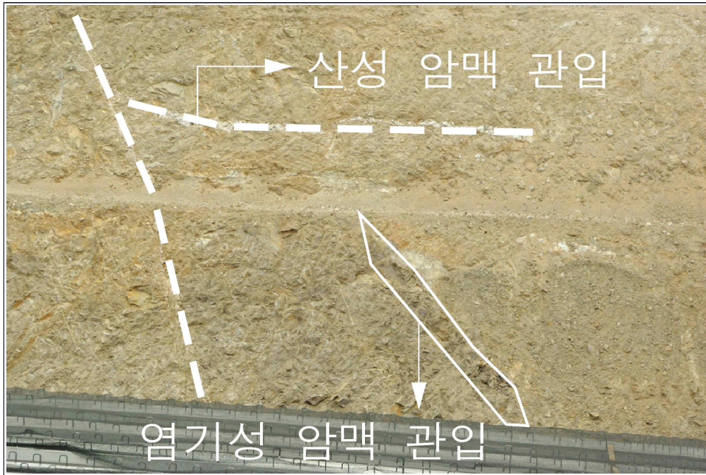
【그림 11】 암맥 관입
