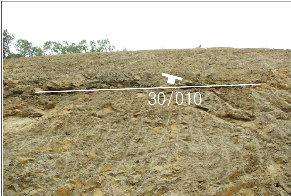
【그림 26】 C 영역에 발달한 불연속면
