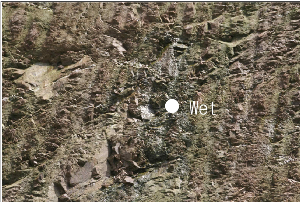
【그림 24】 B 영역 상세사진 (지하수 유출)
