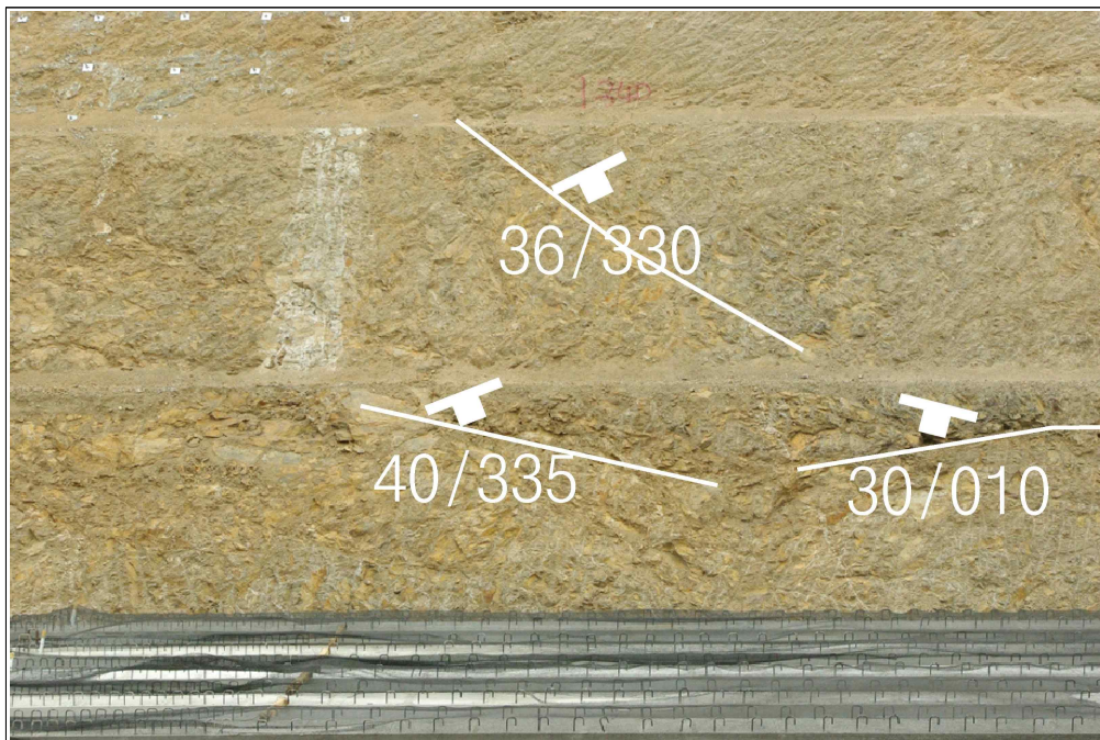
【그림 25】 C 영역에 발달한 불연속면
