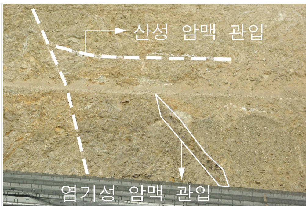
【그림 29】 C 영역 상세사진 (암맥 관입)
