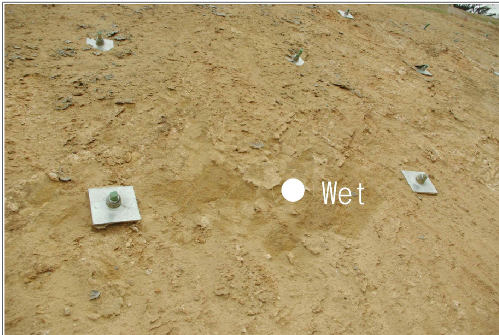
【그림 30】 C 영역 상세사진 (지하수 유출)
