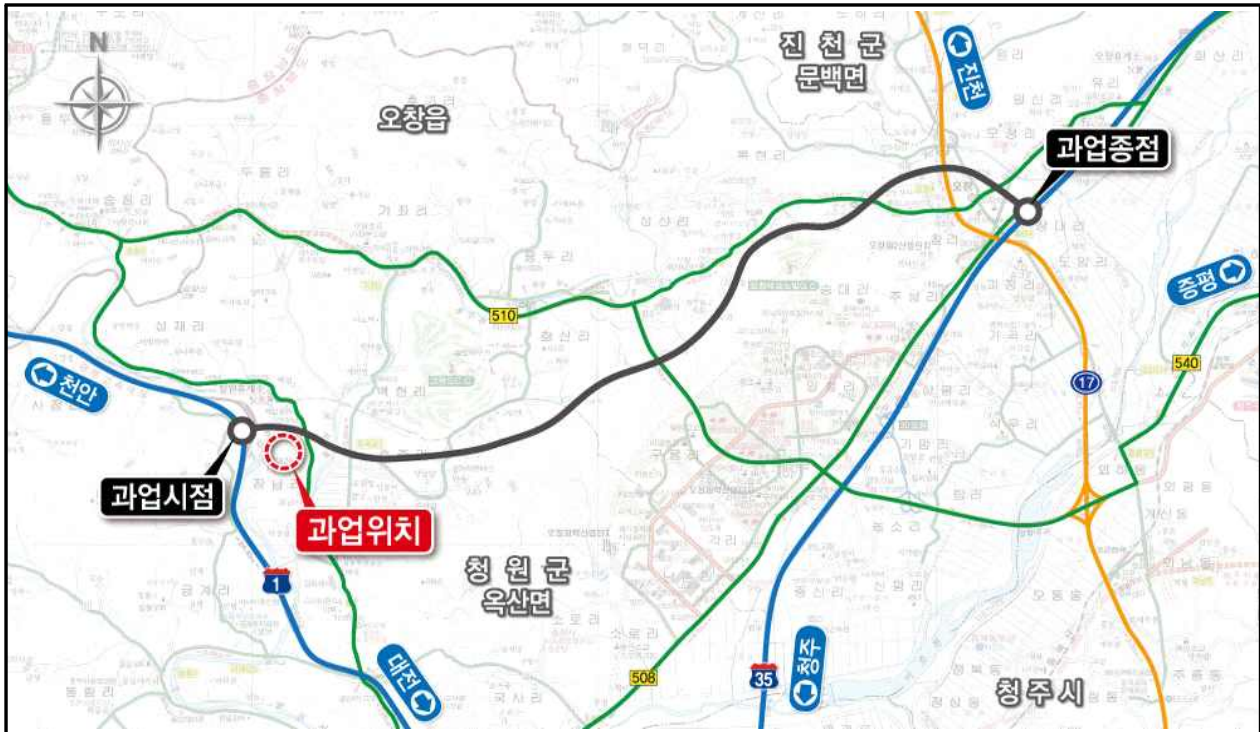
【그림 1】 조사대상 깎기비탈면 위치도
