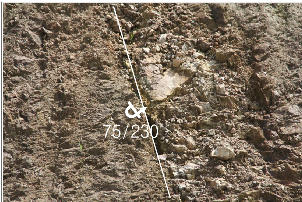
【그림 18】 B 영역에 발달한 불연속면
