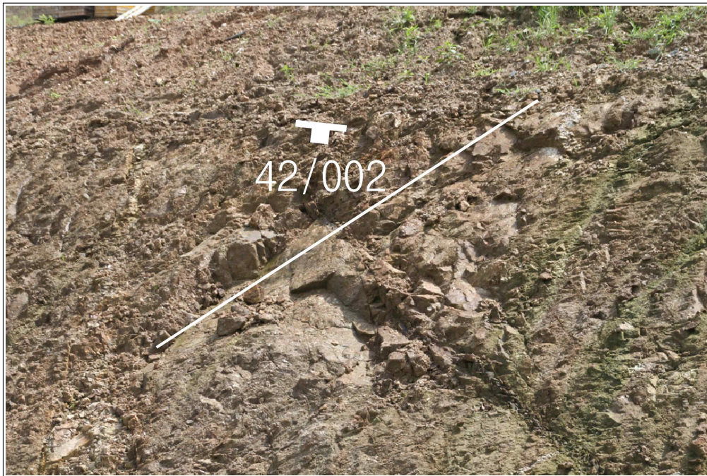
【그림 19】 B 영역에 발달한 불연속면
