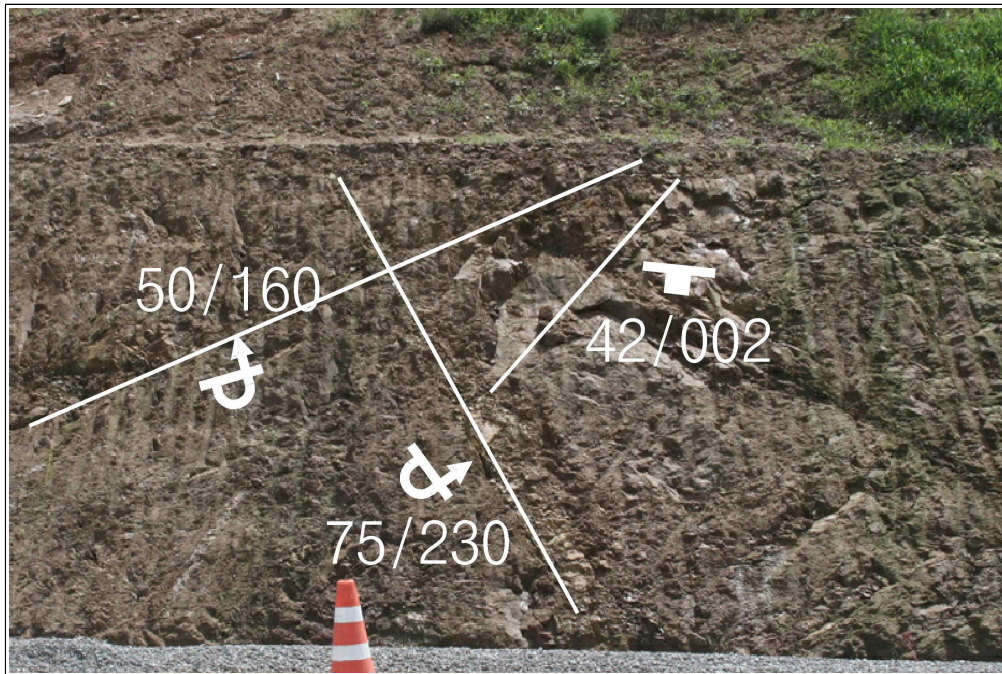
【그림 17】 B 영역에 발달한 불연속면
